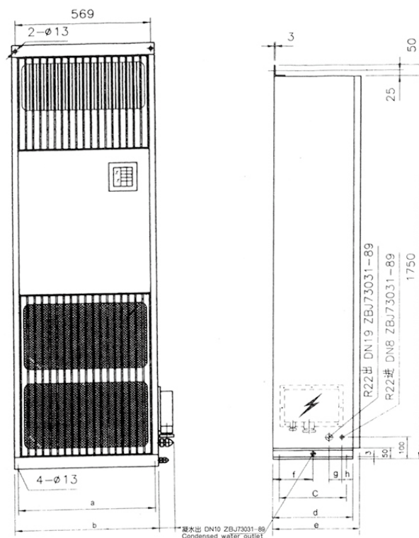
室内机 Indoor unit
